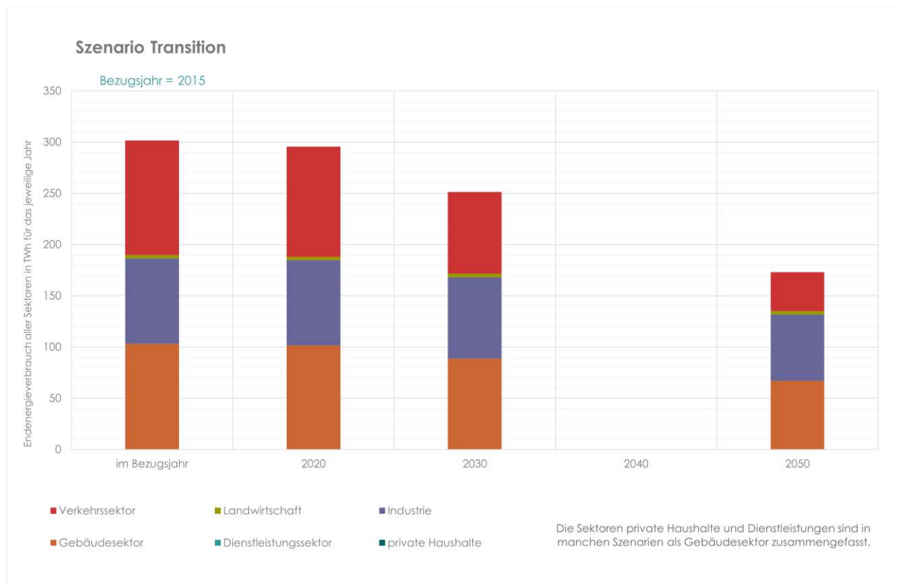
Abbildung 3: Entwicklung des Endenergieverbrauchs im Szenario Transition
